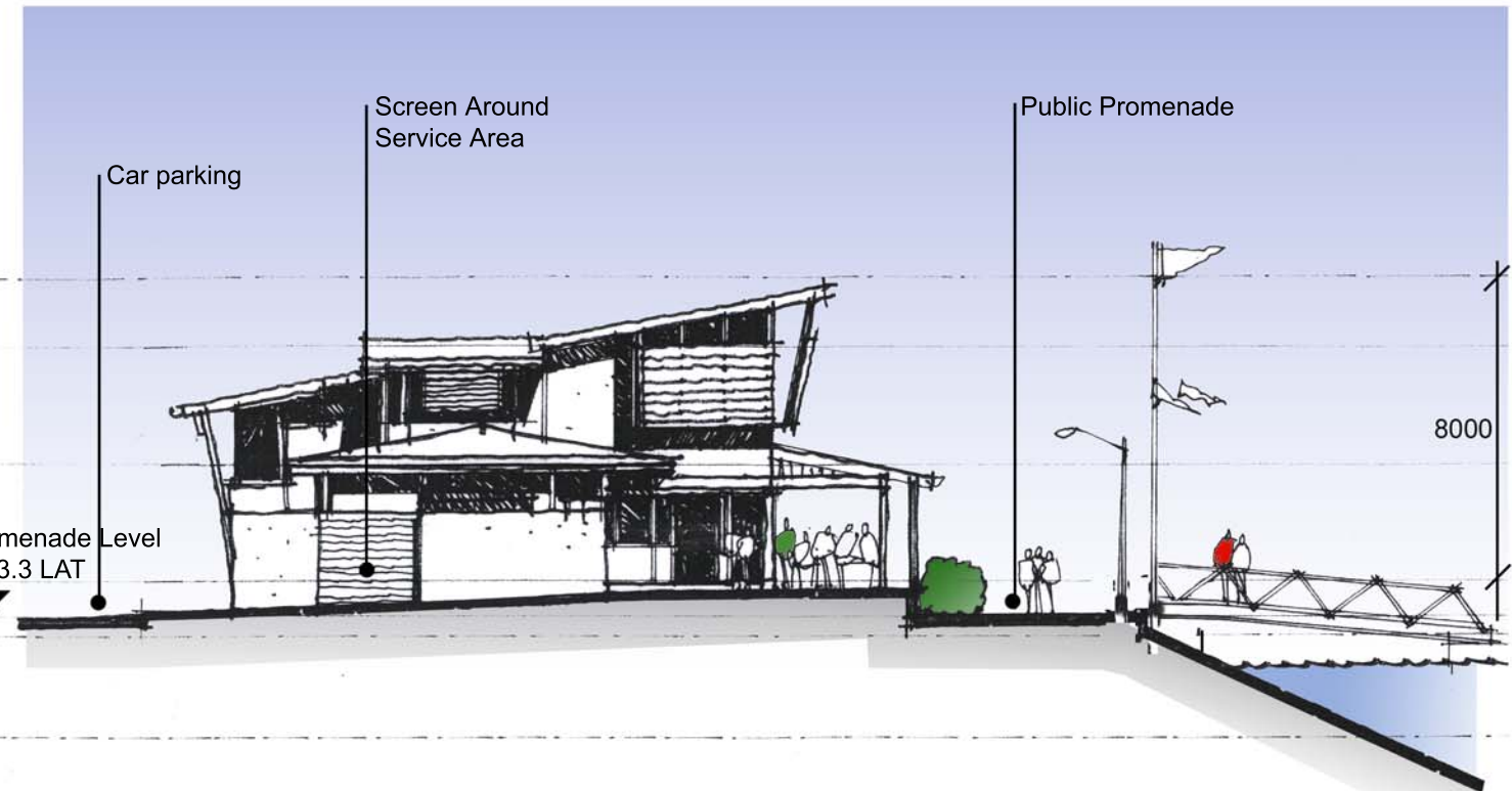
YACHT CLUB ELEVATION E10
