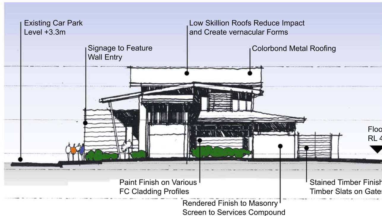
YACHT CLUB ELEVATION E11
